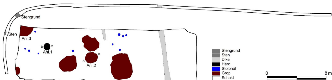
Figur 3. Schaktplan med de två schakten för tillbyggnaden och fjärrvärmen.
